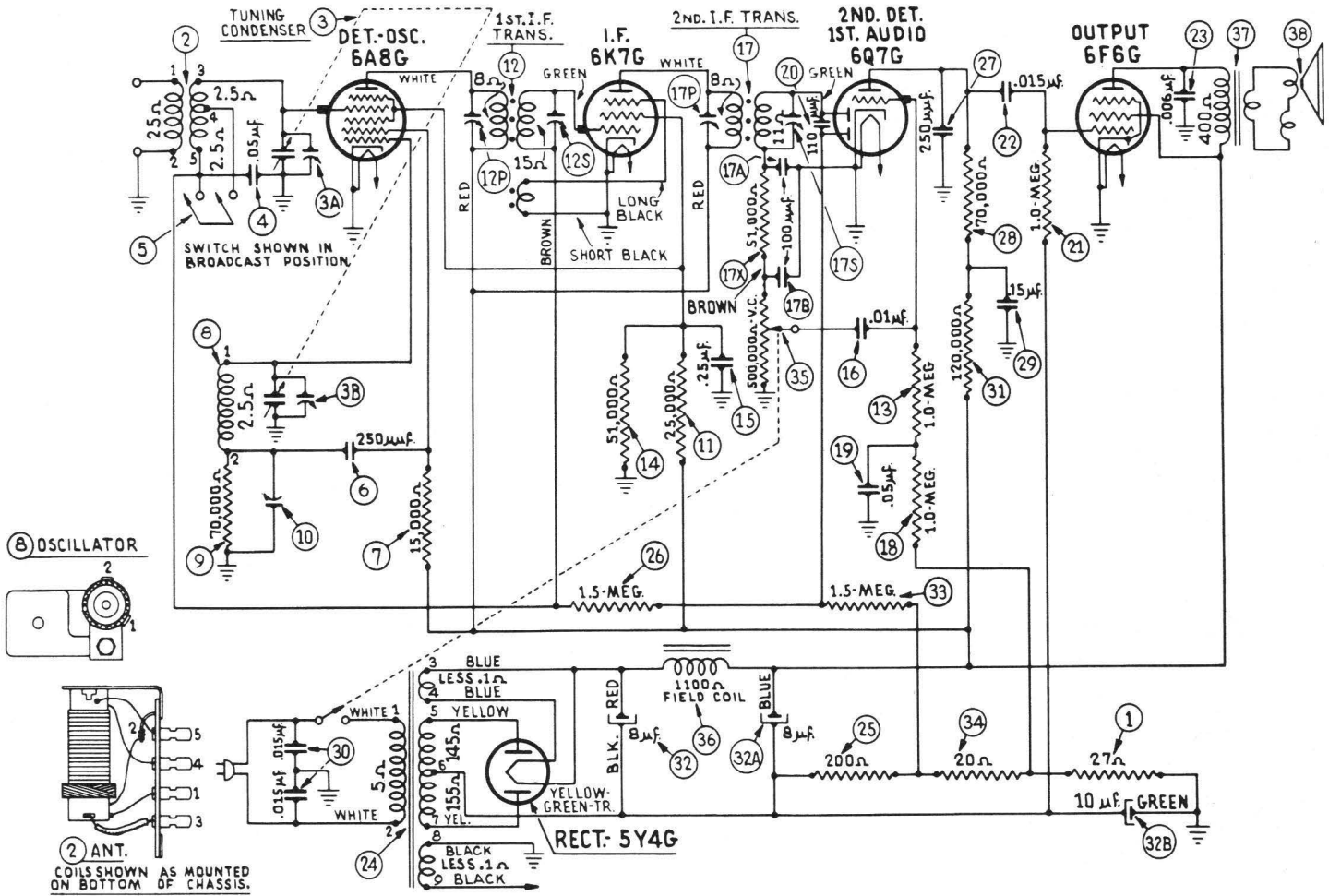
Fig. 4. Schematic Diagram—Model 37-62
